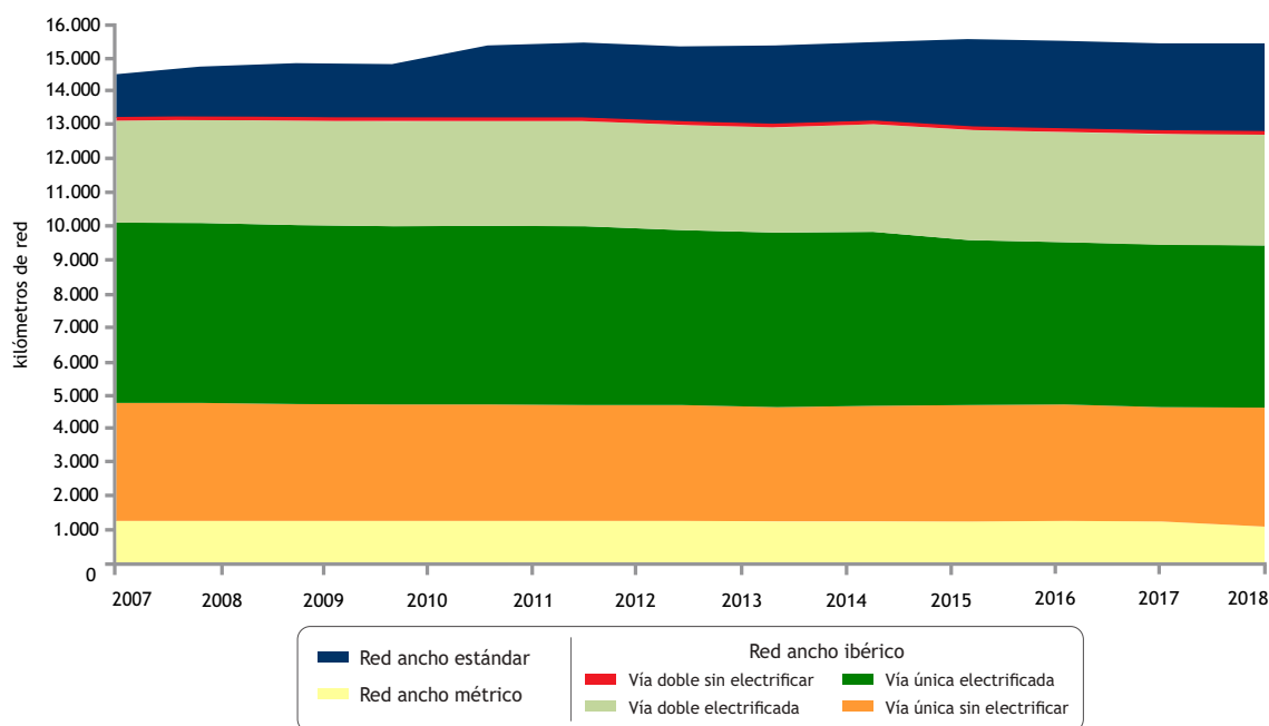
Longitud de las redes según características de la vía en la red gestionada por Adif (2007-2018)
